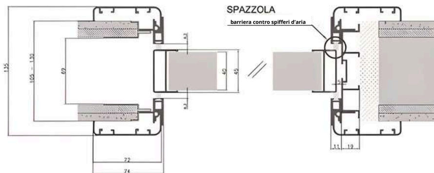
SEZ. A - A
